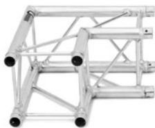
ALUTRUSS DECOLOCK DQ4-PAC21 2-way corner 90° No. 60301734.....4.6 kg
