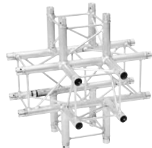
ALUTRUSS DECOLOCK DQ4-PAT51 5-way corner No. 60301768.....5.5 kg
