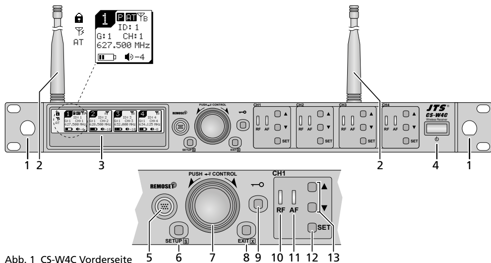
Abb. 1 CS-W4C Vorderseite
