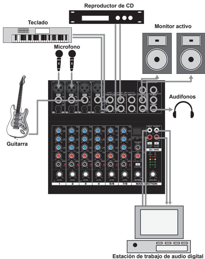
Fig. 3.1: la consola en un estudio de grabación
