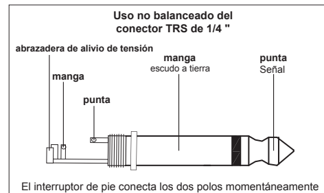
Fig. 4.2: conector estéreo de 1/4 "
