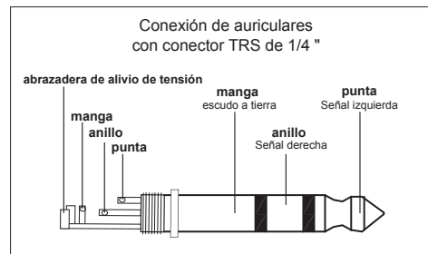
Fig. 4.4: enchufe estéreo para conexión de auriculares
