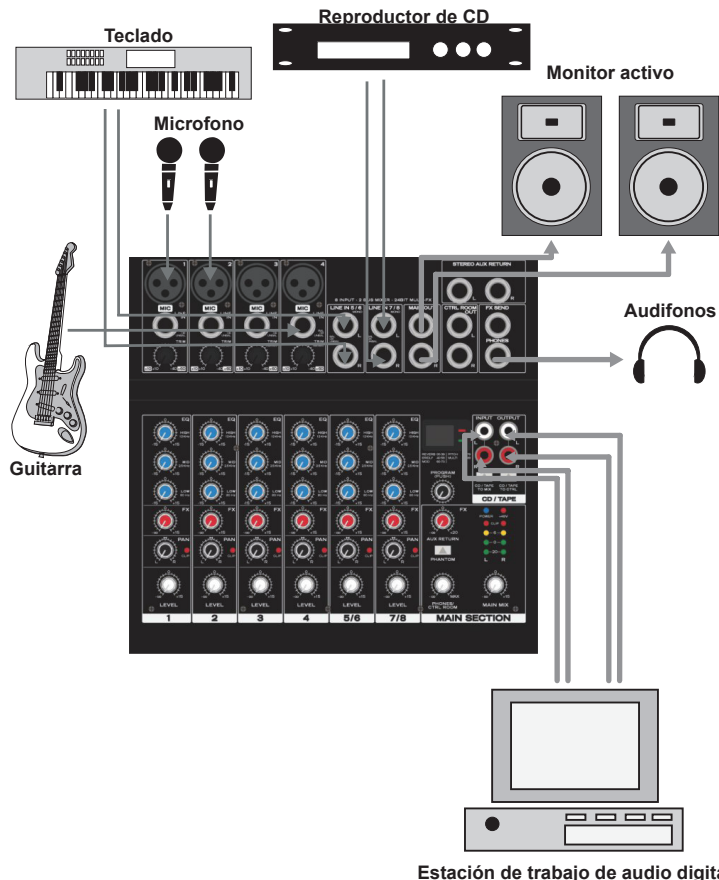
Fig. 3.2: Aplicación en vivo de la consola
