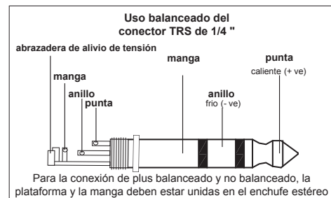
Fig. 4.3: conector estéreo de 1/4 "
